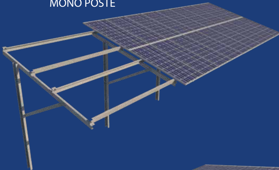
MONO POSTE
